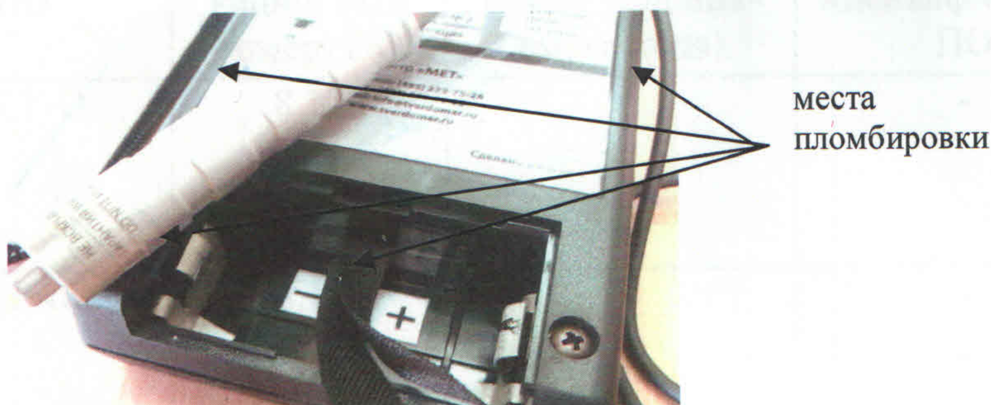
Рисунок 2 - Схема пломбировки твердомера.
