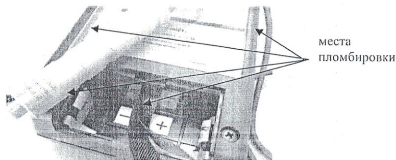
Рисунок 2 - Схема пломбировки твердомера.
